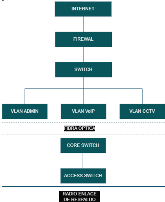
Diagrama lógico de arquitectura.
